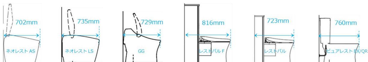
図3. さまざまな便器の種類と奥行寸法の比較
