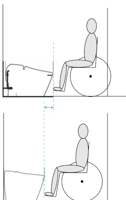
図4. 便器寸法とトイレの広さ
