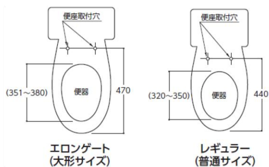
図1. 便器のサイズについて
